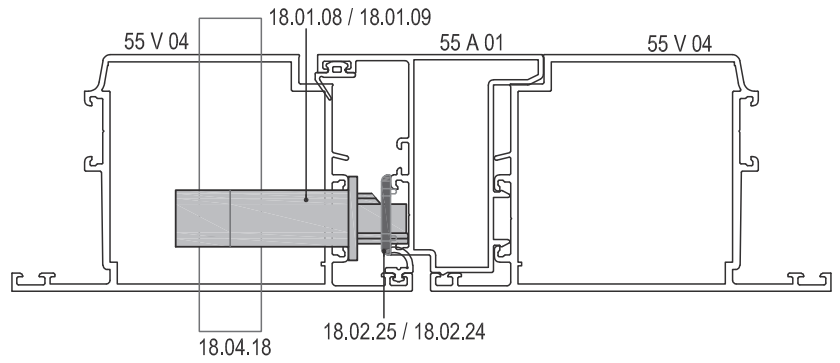
**DIŞA AÇILIM BİNLİ ORTA BİRLEŞİM DETAYI İÇİN (55 A 01) **OUTWARD OPENING FLUSH DOOR ADAPTER DETAIL (55 A 01)
